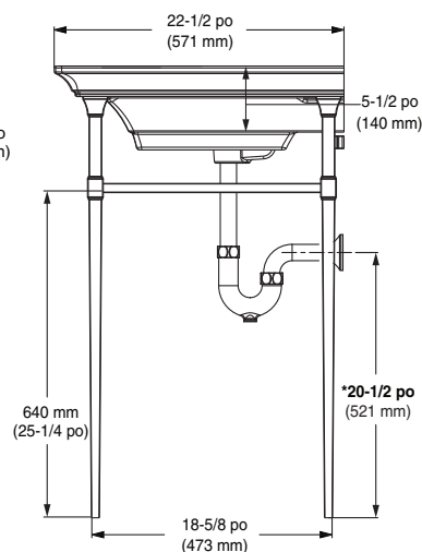
LAVABO SUR COLONNE AVEC CONSOLE
