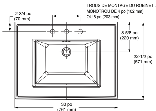
LAVABO SUR COLONNE VUE DE DESSUS
