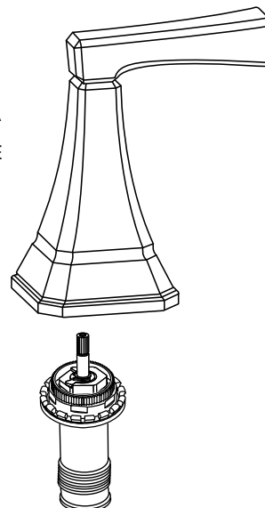
M970479-0070A ENSEMBLE D'ASSEMBLAGE DE TIGE
