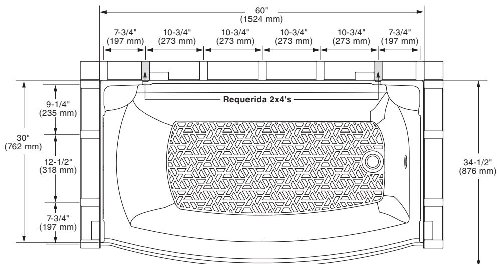
Instalación de montantes en alcoba al instalar el sistema de pared de ducha Ovation
