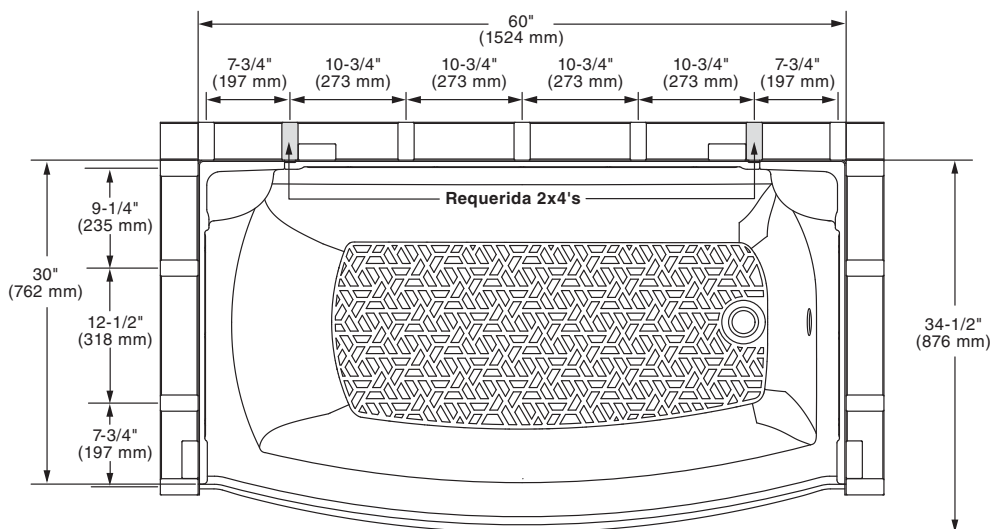
Instalación de montantes en alcoba al instalar el sistema de pared de ducha Elevate
